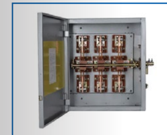
Cầu dao hộp 3 pha 4 cực 300A
