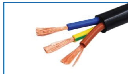
Dây điện 3 lõi VCmt-3x1.5 mm 2 – 300/500V
